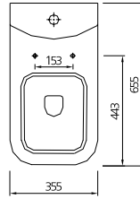
71110340xx Babel Klozet [Duvara Sırt] [Taharet Delikli] Babel WC Pan [Back to Wall] [With Cleaning Pipe] 71110343xx Babel Klozet [Duvara Sırt] [Taharet Deliksiz] Babel WC Pan [Back to Wall] [Without Cleaning Pipe] 71110400xx : 71110405xx : 71110415xx Babel Rezervuar / Babel Cistern [Altın Çıkış] : [Yandan Çıkış] : [Montaj Delikli] [Bottom Inlet] : [Side Inlet] : [With Assembly Hole] 70110720xx Babel Klozet Kapağı Babel Seat & Cover 70110728xx Babel Yavaş Kapanan Klozet Kapağı Babel Soft Close Seat & Cover
